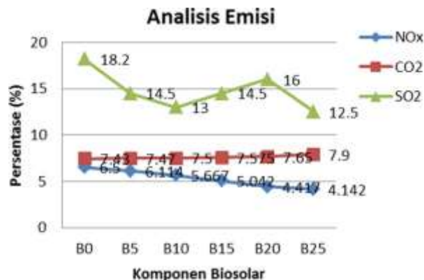
Gambar 8. Hasil Analisis Emisi Gas Buang
