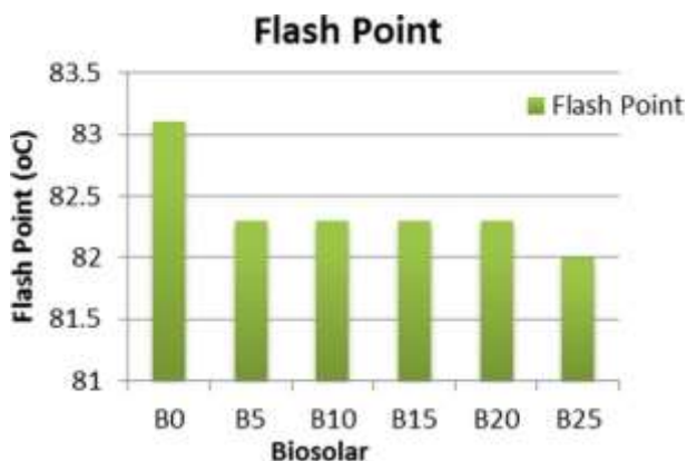
Gambar 7. Pengaruh Biosolar Terhadap Flash Point
