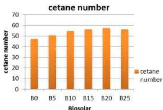
Gambar 6. Pengaruh Biosolar Terhadap Cetane Number
