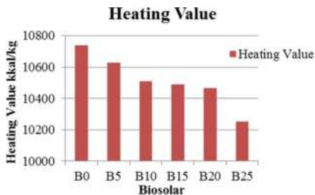
Gambar 5. Pengaruh Biosolar Terhadap Heating Value
